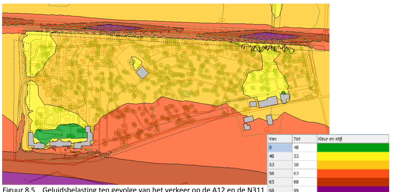
Figuur 8.5 Geluidsbelasting ten gevolge van het verkeer op de A12 en de N311 en afscherming van 9 m hoog aan de A12 zijde (inclusief aftrek)
