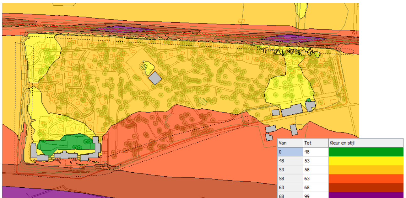
Figuur 4.4 Geluidsbelasting ten gevolge van het verkeer op de A12 en de N311 met scherm langs N311 en afscherming van 9 meter hoog aan de A12 zijde (inclusief aftrek)
