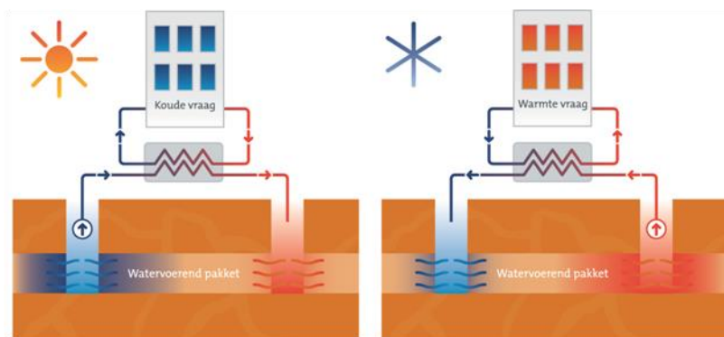
Figuur 2.1 | Principe van een open bodemenergiesysteem
