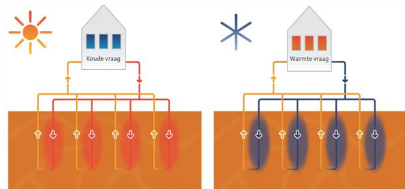
Figuur 2.2 | Principe van een gesloten bodemenergiesysteem
